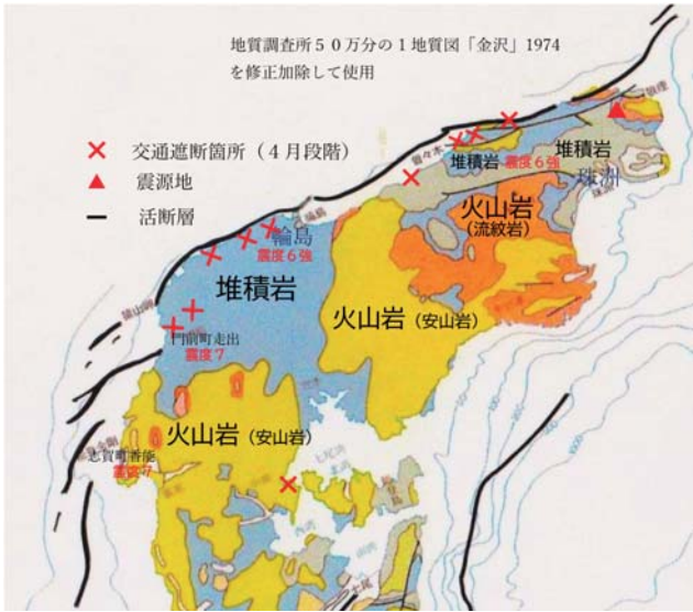
図1「能登半島北部の地質図」
